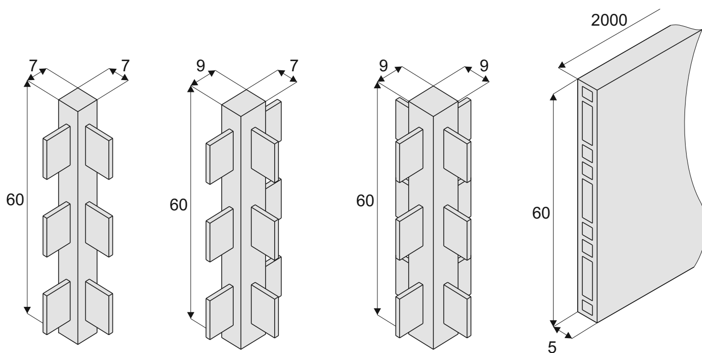
Łącznik dwustronny
