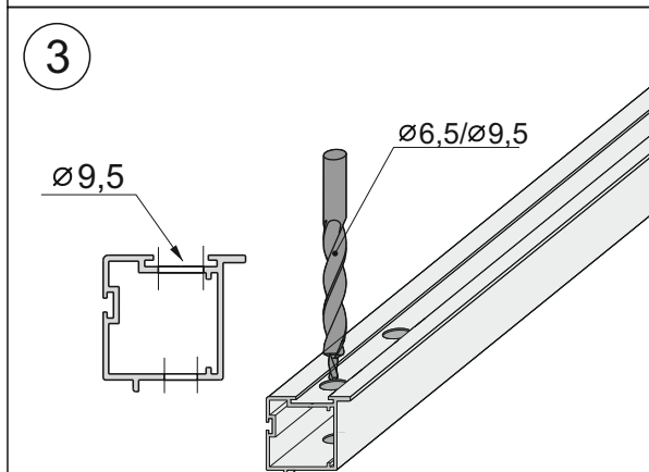
otwory \varnothing 6,5 w gnieździe na szczotkę rozwiercić wiertłem \varnothing 9,5 (zalecane wiertło stopniowe)
