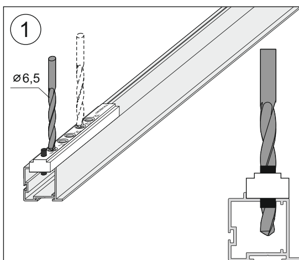
System GEMINI 4 - otwory 9 i 42 mm System EDEN 4 - otwory 21 i 55 mm
