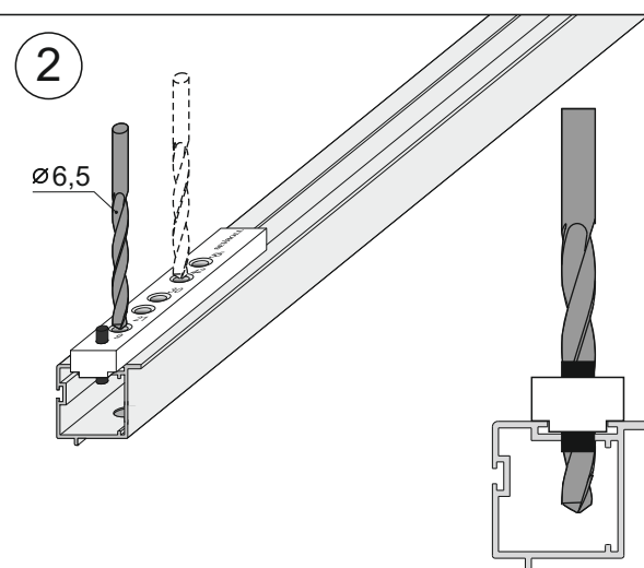
System GEMINI 4 - otwory 9 i 42 mm System EDEN 4 - otwory 21 i 55 mm
