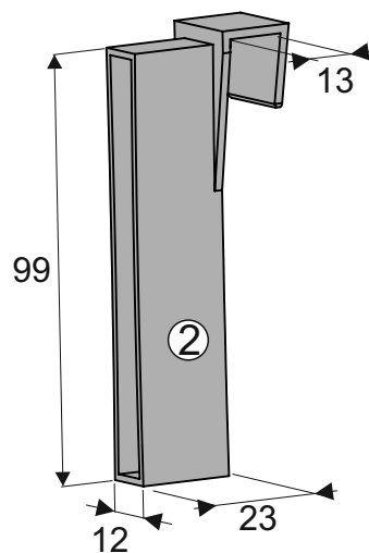
Adapter montażowy MIX do listwy poprzecznej dla szuflad SLIM
