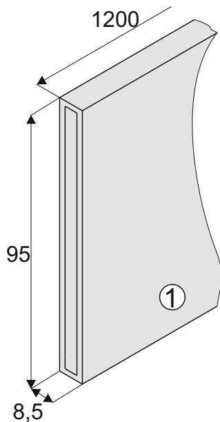
Listwa poprzeczna MIX do podziału szuflad SLIM
