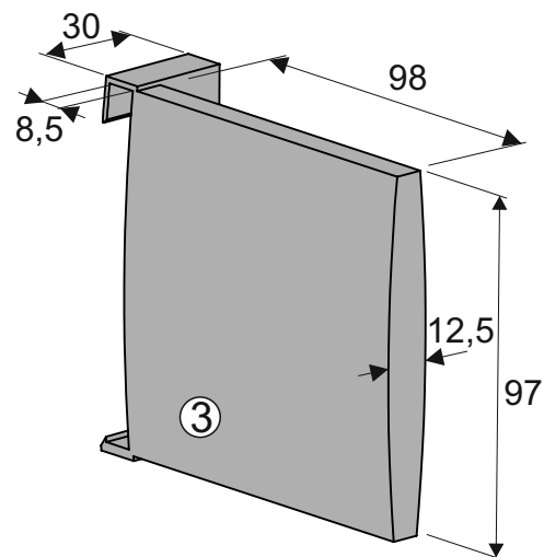
Przegródka MIX do listwy poprzecznej dla szuflad SLIM
