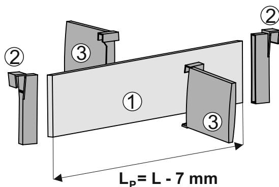
Adapter montażowy MIX do listwy poprzecznej dla szuflad SLIM
