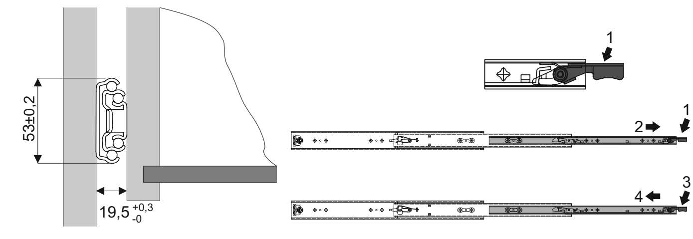
Wymiary prowadnic
