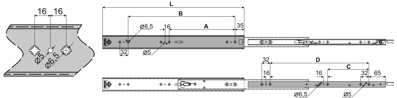
Mocowanie prowadnic do korpusu
