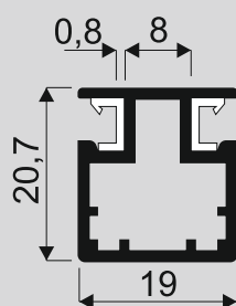
Łącznik do ramek S01 i S05
