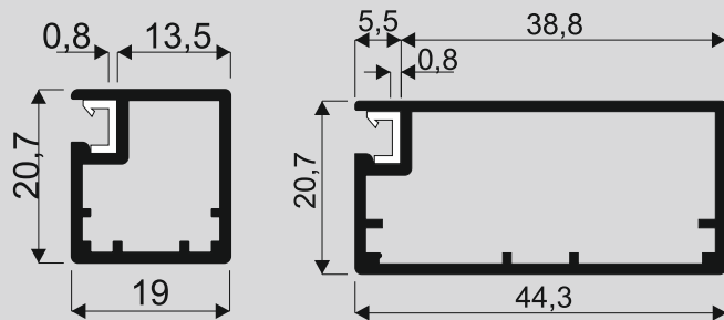
Ramka S01 II
