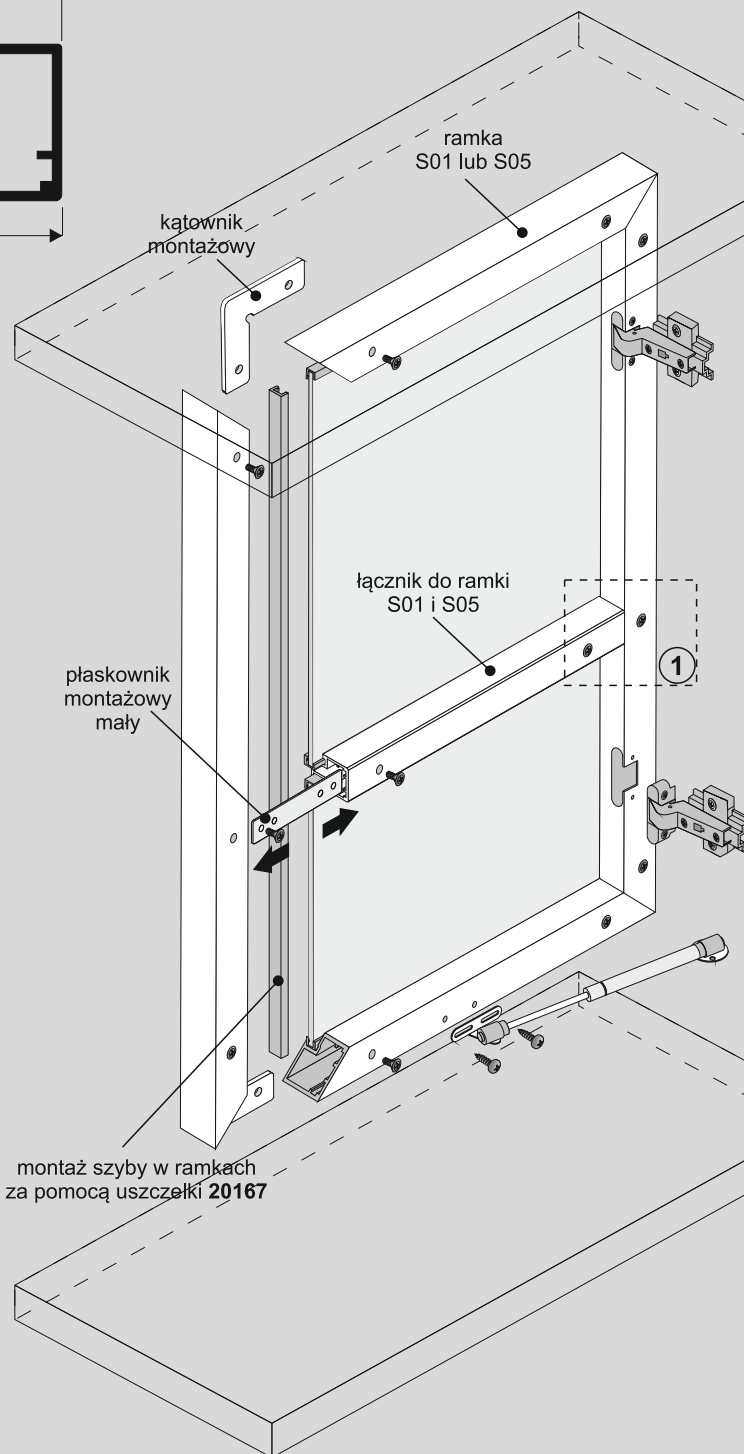
Łącznik do ramek S01 i S05
