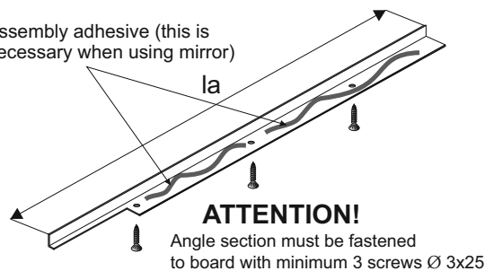
Angle section MINI 11 mm x 17 mm (board)
